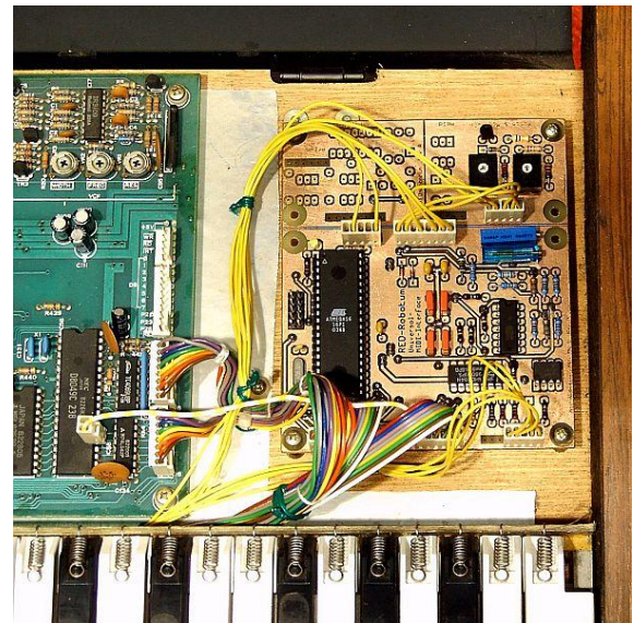
Das MIDI-for-Vintage-Synth-Interface im Roland Juno-6
