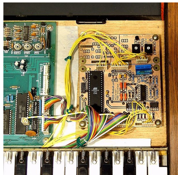
Das MIDI-for-Vintage-Synth-Interface im Roland Juno-6
